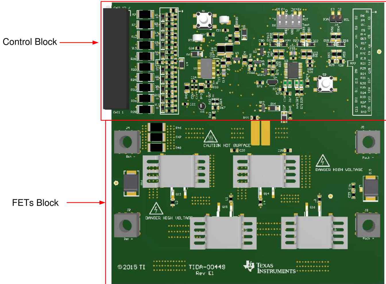
图 29. 布局方框图
