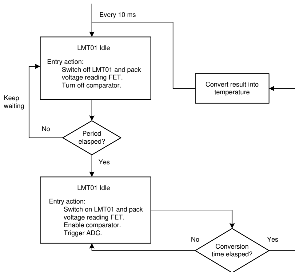
图 4. LMT01 流程图
