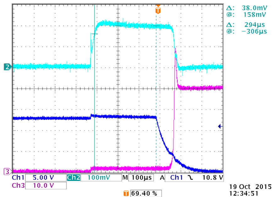
图 18. 短路保护
