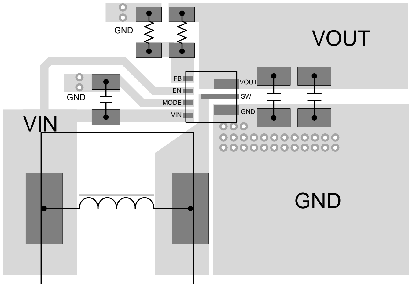
图 29. Layout Example
