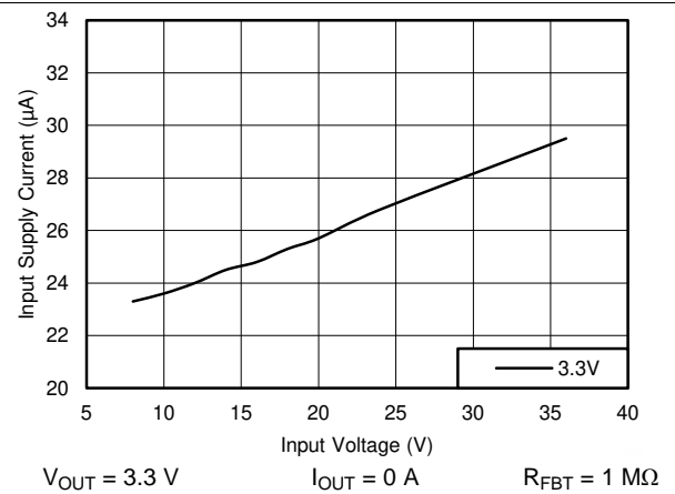
图 45. Input Supply Current
