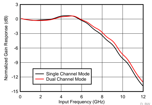
ADC12DJ3200 测量的输入带宽
